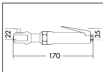
Διαστάσεις του μοντέλου 1/4" και του μοντέλου 3/8"
